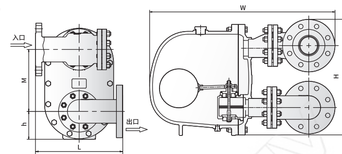
SFT80A Dimension Table
